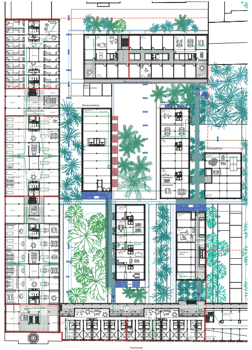
Plan 2. OG | 1:250
