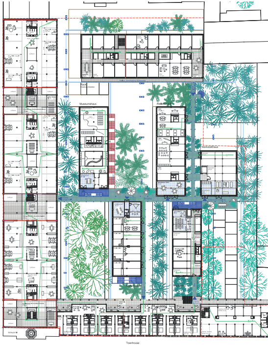
Plan 1. OG | 1:250
